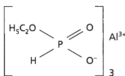
Fosetyl aluminum
