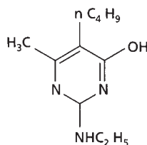
Ethirimol (2-aminopyrimidine)
